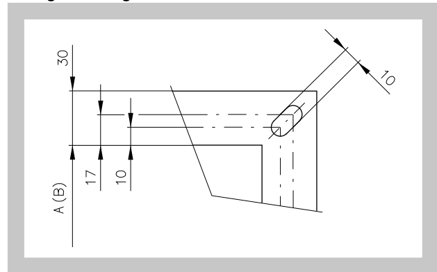
Fig. 5 Flanges
